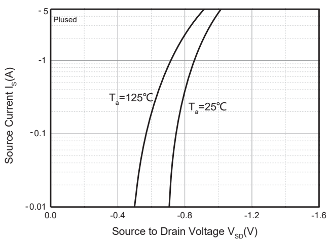
I_S - V_{SD}
