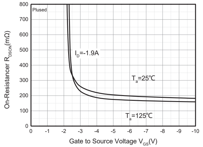
R_{DS(ON)} - V_{GS}
