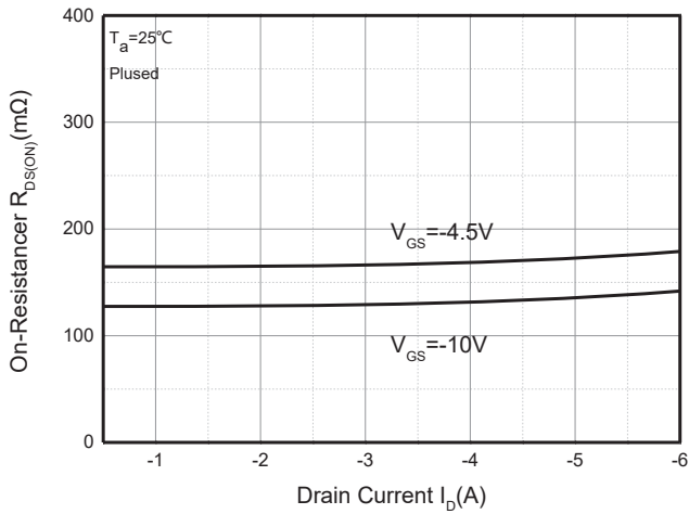
R_{DS(ON)} - I_D
